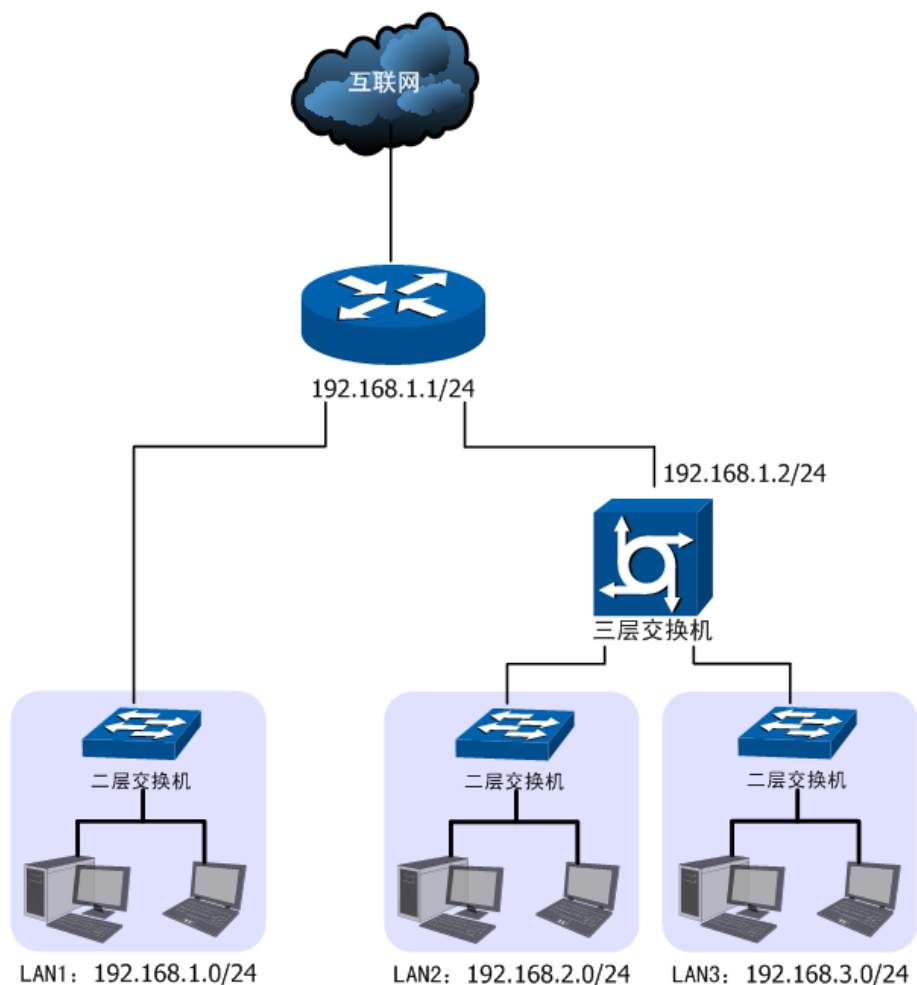
图 4-48 静态路由功能组网应用
