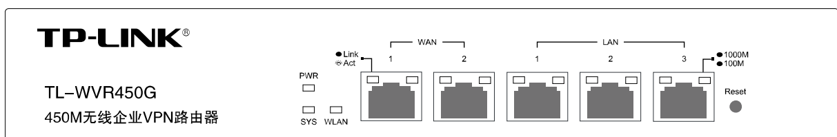
图 2-1 TL-WVR450G前面板示意图
