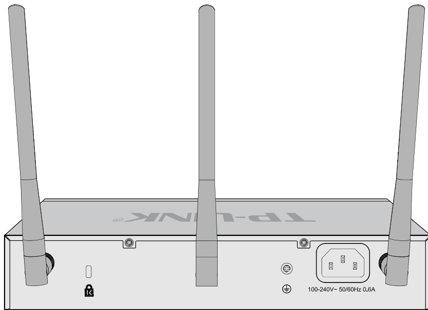
图 2-2 TL-WVR450G后面板示意图
