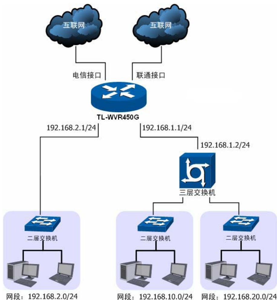
图 4-34 NAPT功能组网应用
